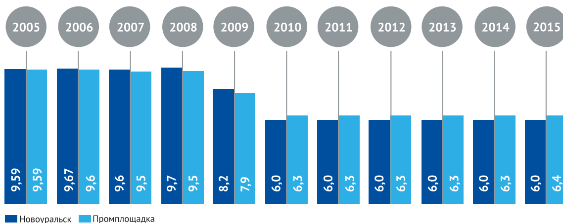
Диаграмма 1. Мощность экспозиционной дозы, мкР/ч
