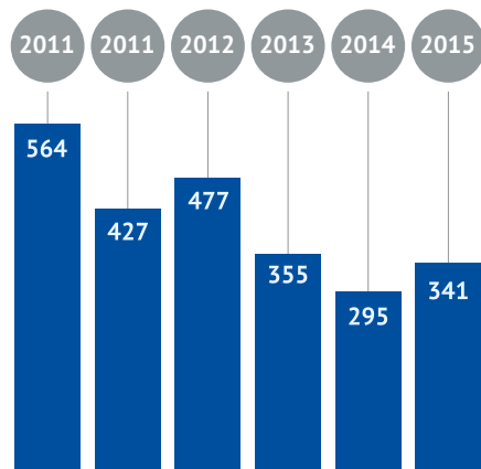
Диаграмма 5. Образование ТРО, м³
