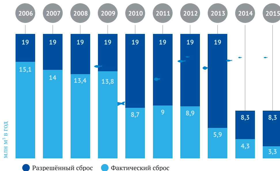
Диаграмма 2. Объём сточных вод
