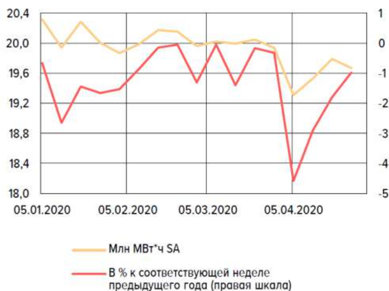
ПОТРЕБЛЕНИЕ ЭЛЕКТРОЭНЕРГИИ С ИСКЛЮЧЕНИЕМ ТЕМПЕРАТУРНОГО ФАКТОРА (ЗА НЕДЕЛЮ)
