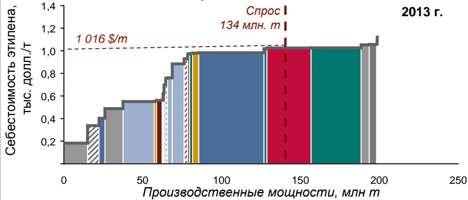
Сравнение конкурентоспособности производственных мощностей этилена
