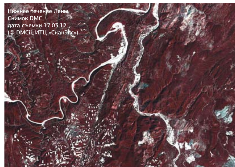
Рена Лена, г. Киренск. Снимок EROS B, дата съёмки 17.03.12 (© ImageSat, ИТЦ «СканЭкс»)
