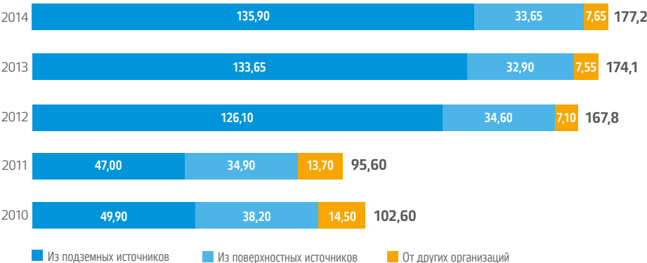
Объем забора и получения воды от различных источников, млн м³
